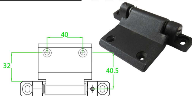
Adjustable Hinge 3019
