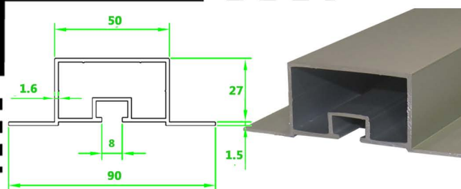
Top Hat 5 cm
