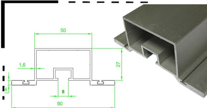
Top Hat 5 cm
