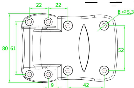
Aluminum hinge
