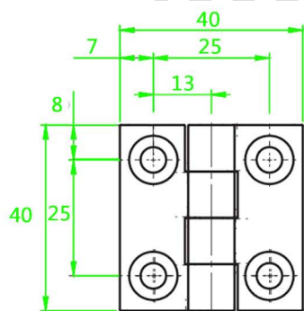
Metal hinge 40*40
